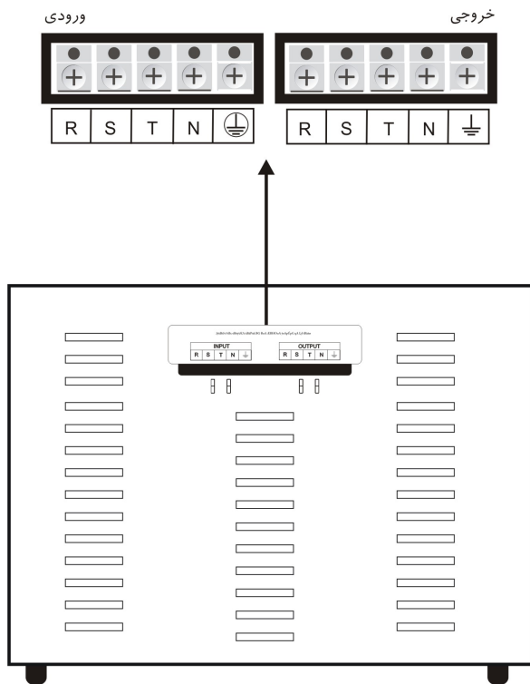
شکل شماره ۲: نمای ترمینال پشت دستگاه
